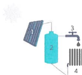
1. Zonnecollector | 2. Opslagvat zonnecollector | 3. Sanitair warm water | 4. Aardvloeren of verwarmingsradiatoren
